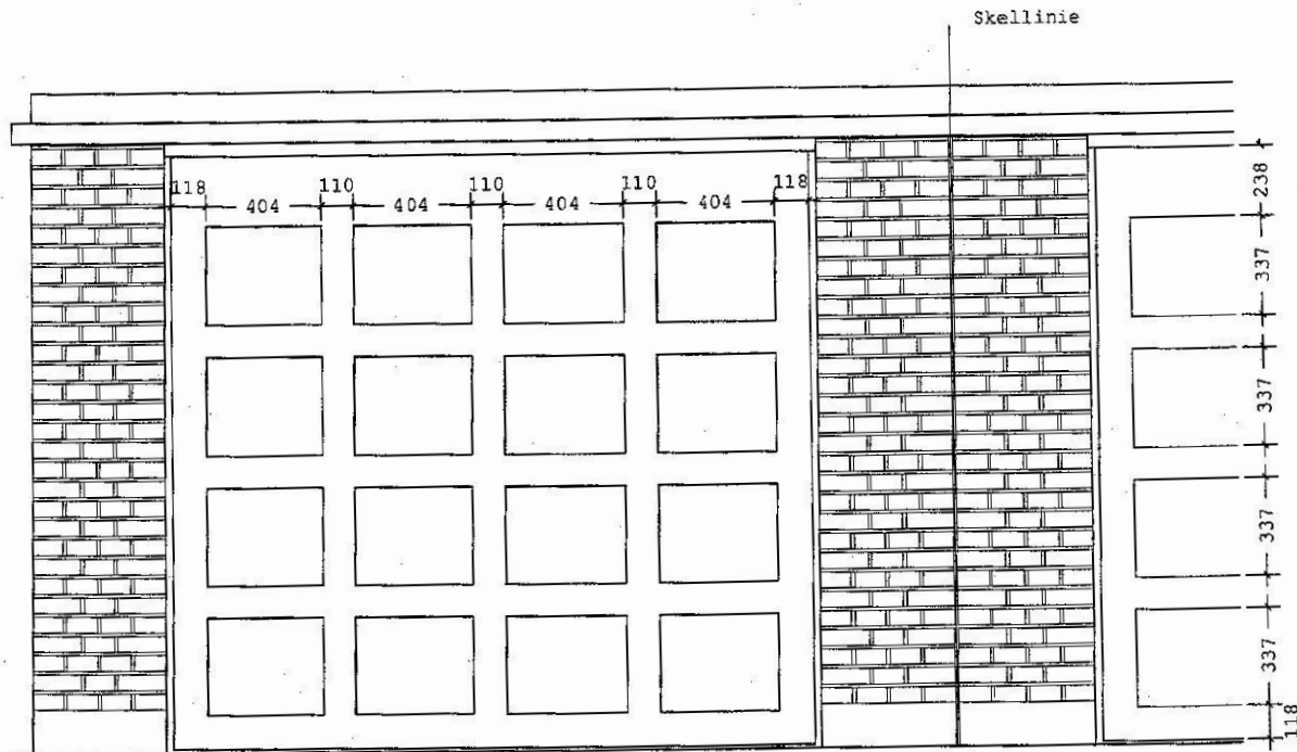
Opstalt af garage mod vejen 1:20
