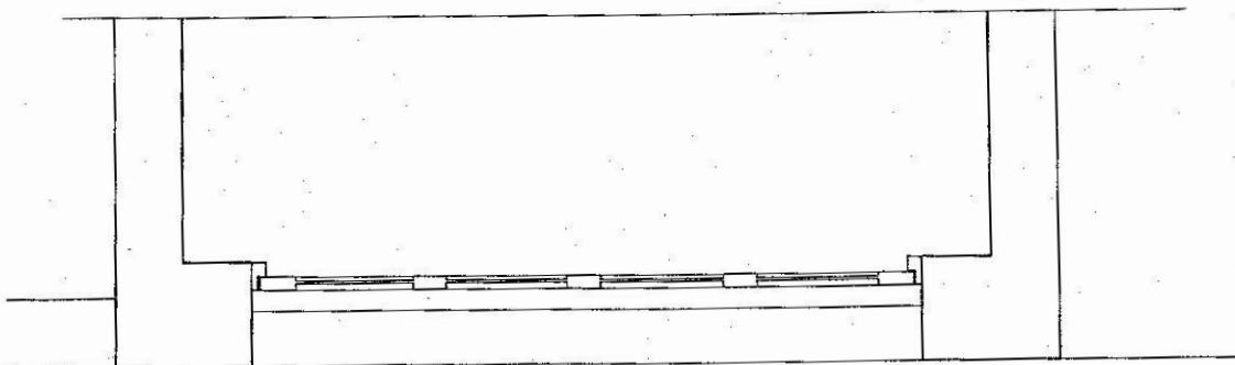
Plan af garageport 1:20
